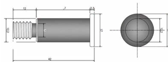
בורג תלייה לחיפוי - נירוסטה 304
