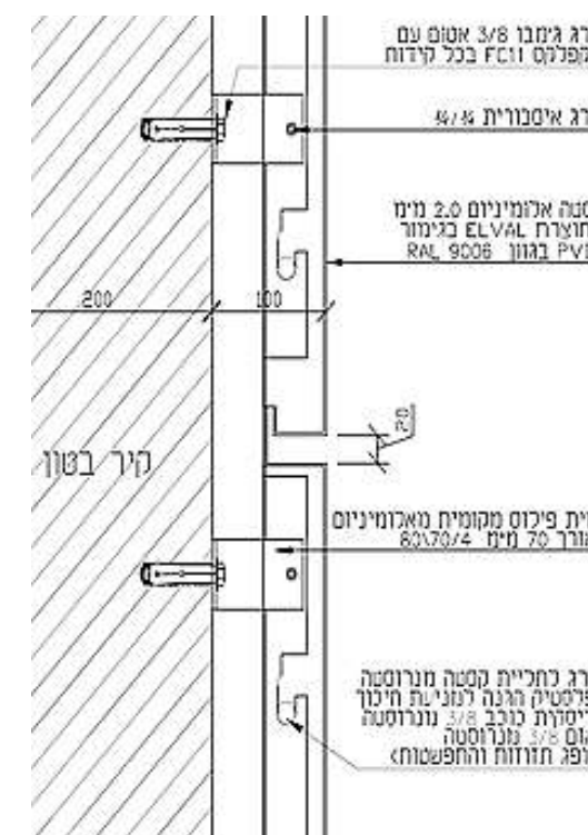
קסטה טיפוסית | מבט פנים
